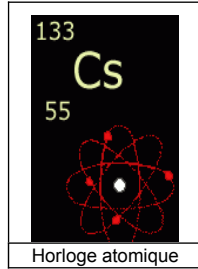
Horloge atomique
